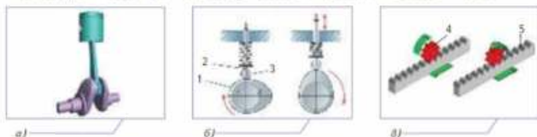
Рис. 4.9. Механизмы передачи и преобразования движений: а — кривошипно-шатунный; б — кулачковый; в — реечный; 1 — кулачок; 2 — шток; 3 — ролик; 4 — колесо; 5 — рейка
